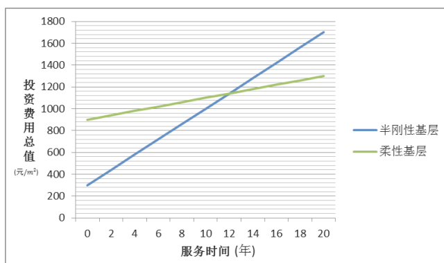
柔性基层与半刚性基层投资费用随时间变化情况
