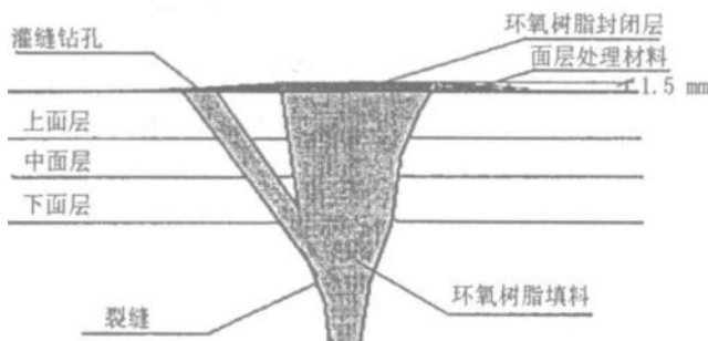
沥青路面裂缝细节图
