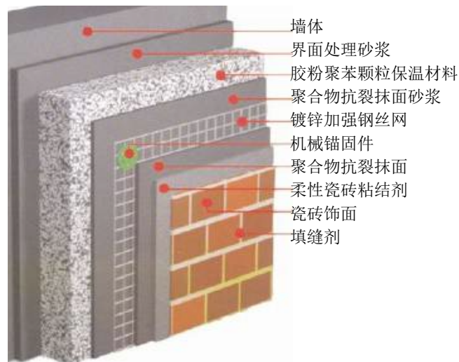
玻化微珠无机保温砂浆墙体
